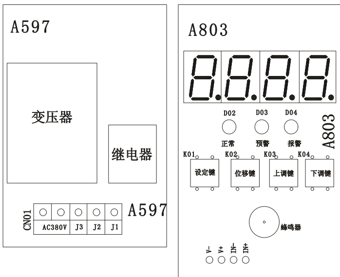
元件布置图
