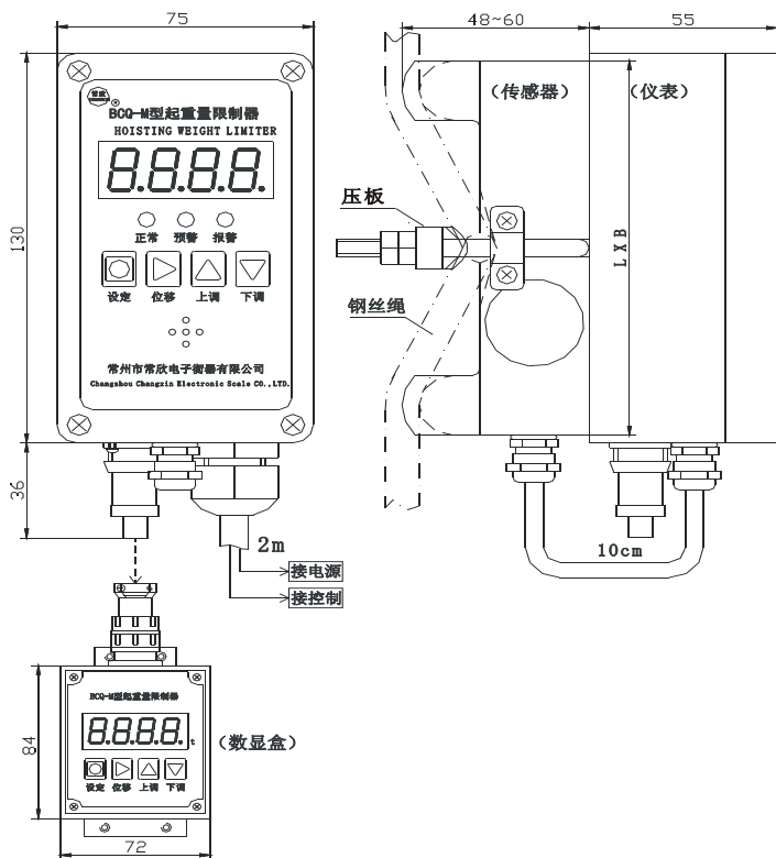
总体连接图
