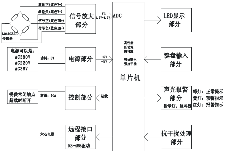
电气原理示意图
